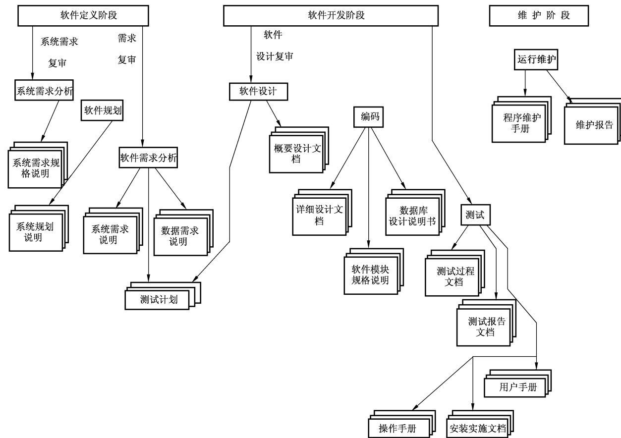
图 B.1 软件生命周期各个阶段应当产生的重要软件文档示意
